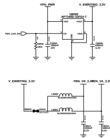
S-PEN LDO
